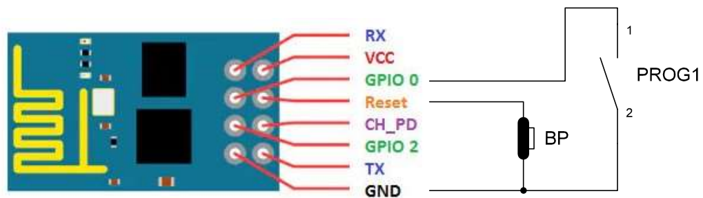
USB / ESP01 câblage ESP01
