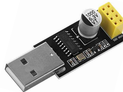
Az-Delivery module USB / ESP01
